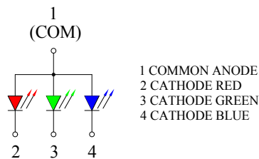
Polarity
