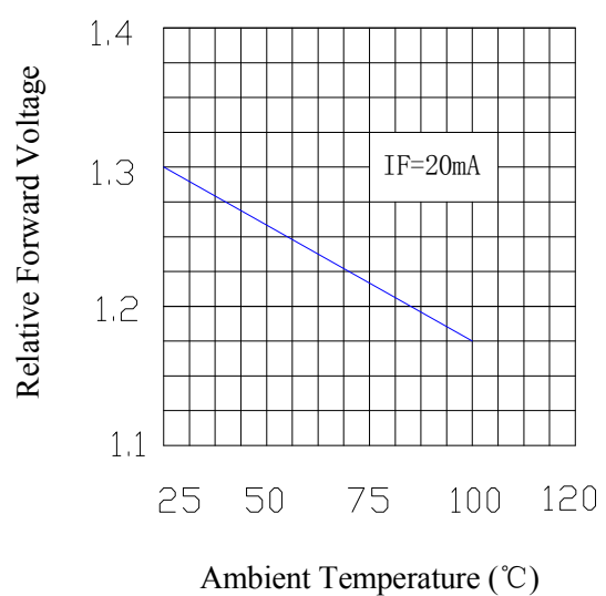
Forward Voltage & Ambient Temperature (°C)
